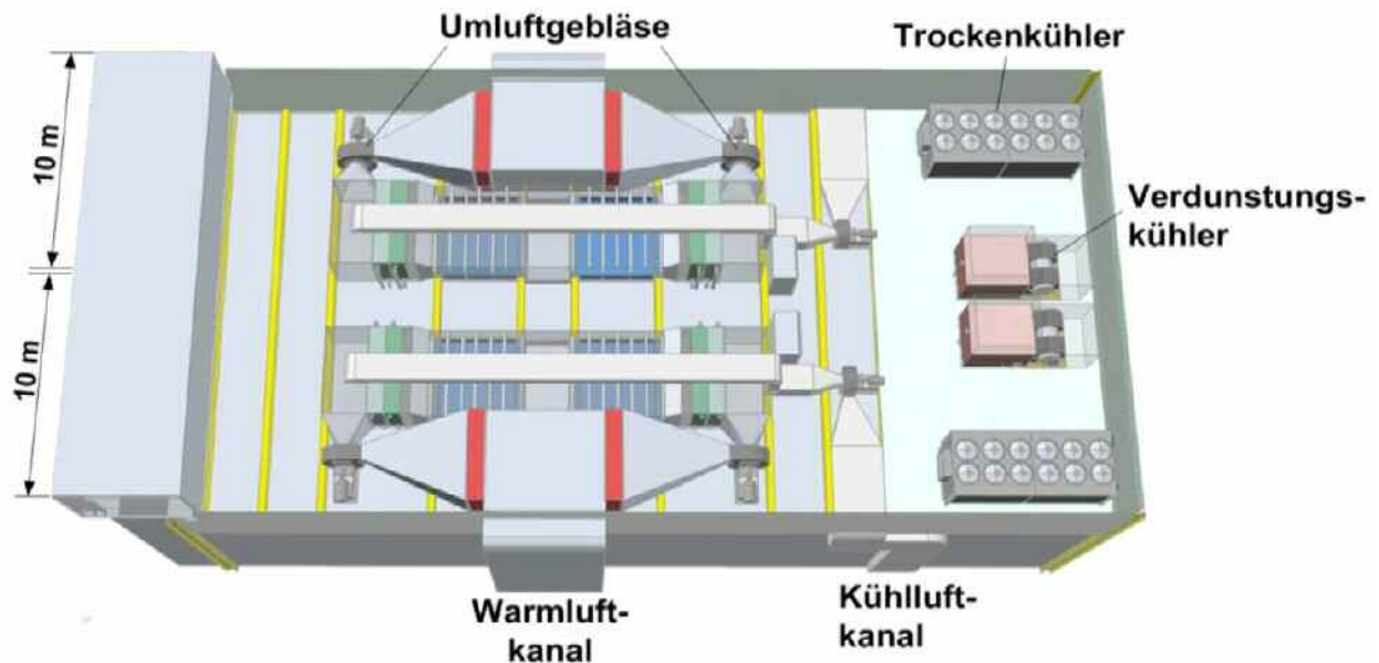
Abbildung 3 Draufsicht des Tunnelrockners
