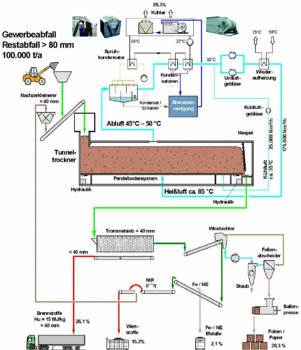
Abbildung 6 Fließbild Tunnelrockner
