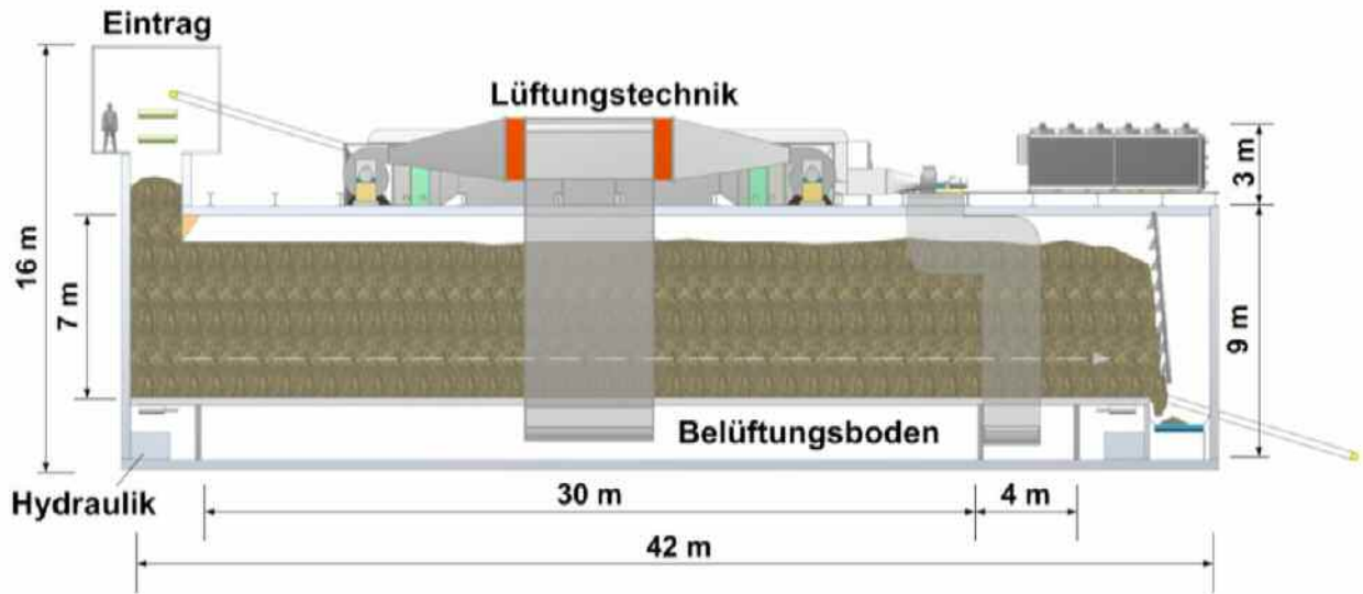
Abbildung 2 Schnitt des Tunnelrockners
